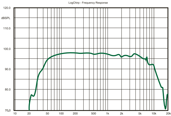
Высокочастотный динамик GAMMA 628C
