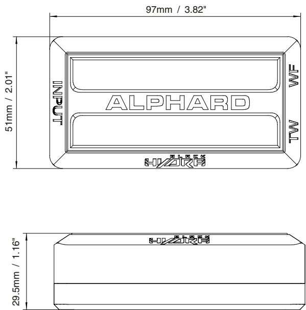
Crossover GAMMA 628C
