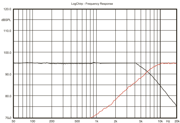
Кроссовер GAMMA 628C
