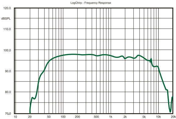
Tweeter GAMMA 628C
